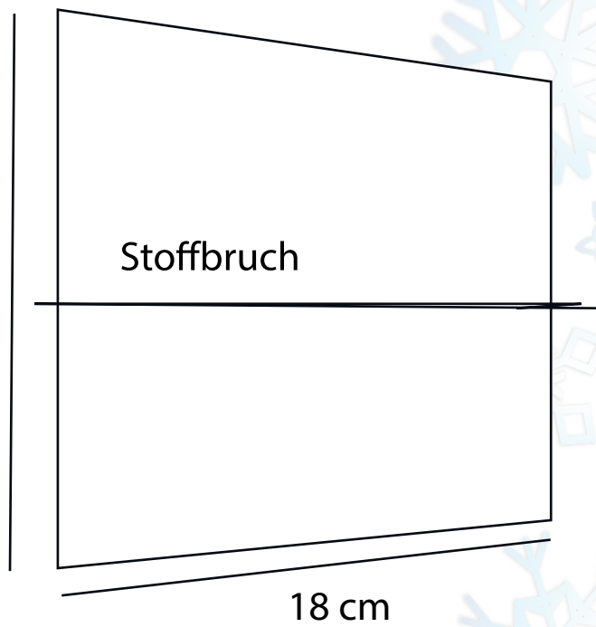
Schnittmuster für Pulswärmer, entsprechend den Zentimeterangaben vergrößern
